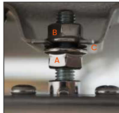
Abb. 07: Wandmontage
