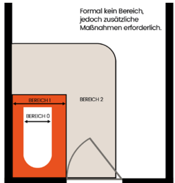
Abb. 02: Montage in Feuchträumen und Badezimmern
